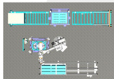
Standardcell uppifrån
